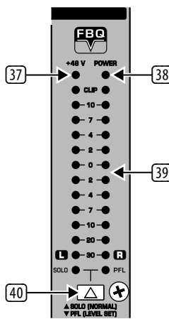
Fig. 2.16: Level meter
