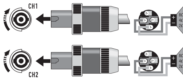
Modo estereofónico, biamplificado o paralelo – Figura 29 –
