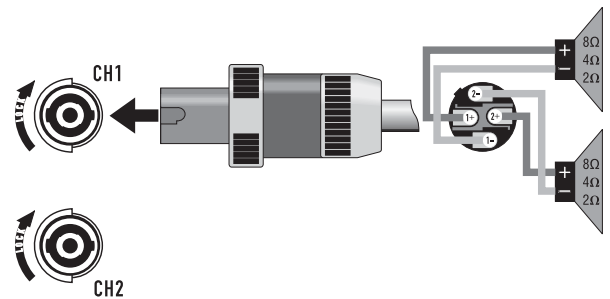
Stéréo, Bi-ampli, ou en mode parallèle – Figure 30 –
