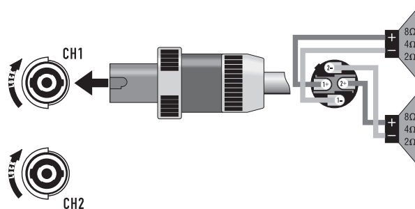
立体声、双放大器或并行模式
