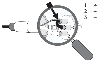
XLR déséquilibrée broche de cavalier 1 à la broche 3
