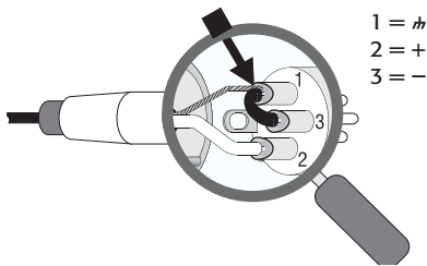
XLR 非平衡跳线引脚 1 至引脚 3
