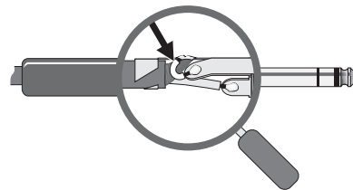
TRS déséquilibré Aucune modification nécessaire
