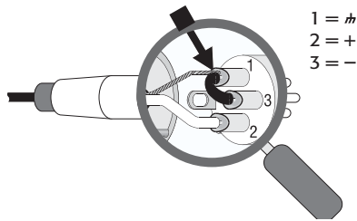
XLR no balanceado Patilla 1 a patilla 3 del puente – Figura 26 –
