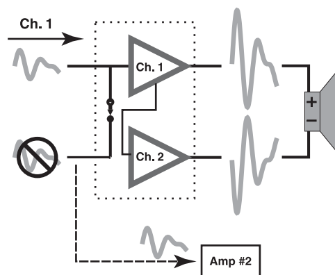
Puede utilizarse para conectar amplificadores adicionales en cadena de margarita – Figura 22 –
