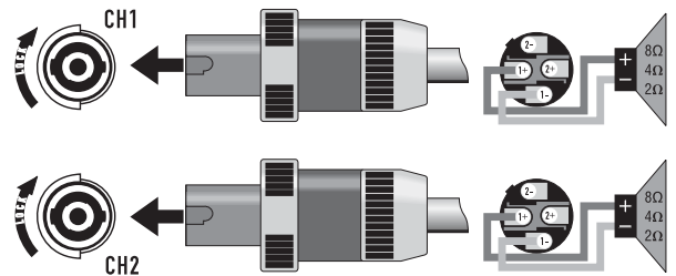
Stéréo, Bi-ampli, ou en mode parallèle – Figure 29 –
