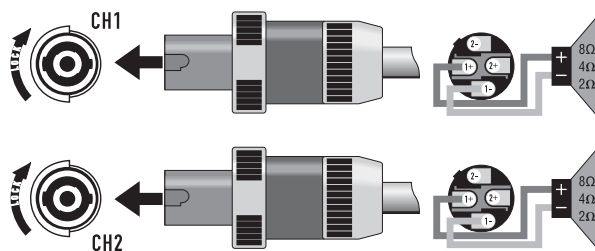
立体声、双放大器或并行模式
