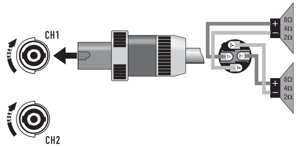
Stereo, Bi-amp, or Parallel Mode – Abbildung 30 –
