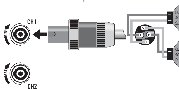
Modo estereofónico, biamplificado o paralelo – Figura 30 –
