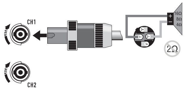
Bridge Mono Mode – Abbildung 31 –
