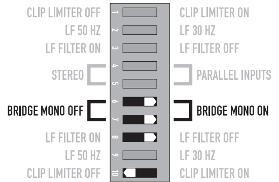
Réglages Canal 2, 8 et 10 commutateurs sont désactivés.
