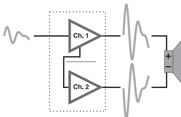
Canal 1 entrada, Canal 2 entrada no utilizado – Figura 21 –
