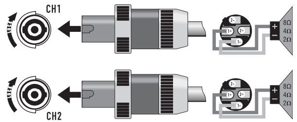
Stereo, Bi-amp, or Parallel Mode – Abbildung 29 –
