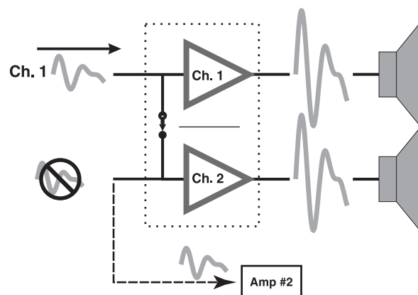
可用于菊链其他放大器
