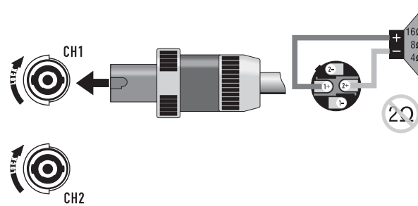
Modo monofónico puenteado – Figura 31 –
