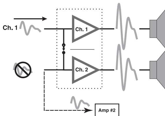
Peut servir au branchement en guirlande d'amplificateurs supplémentaires
