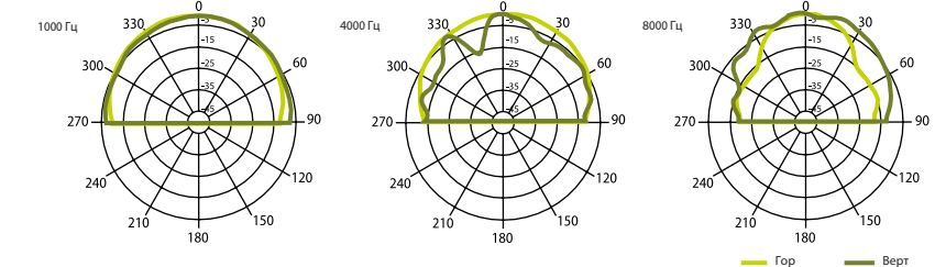
Горизонтальная/вертикальная диаграммы направленности
