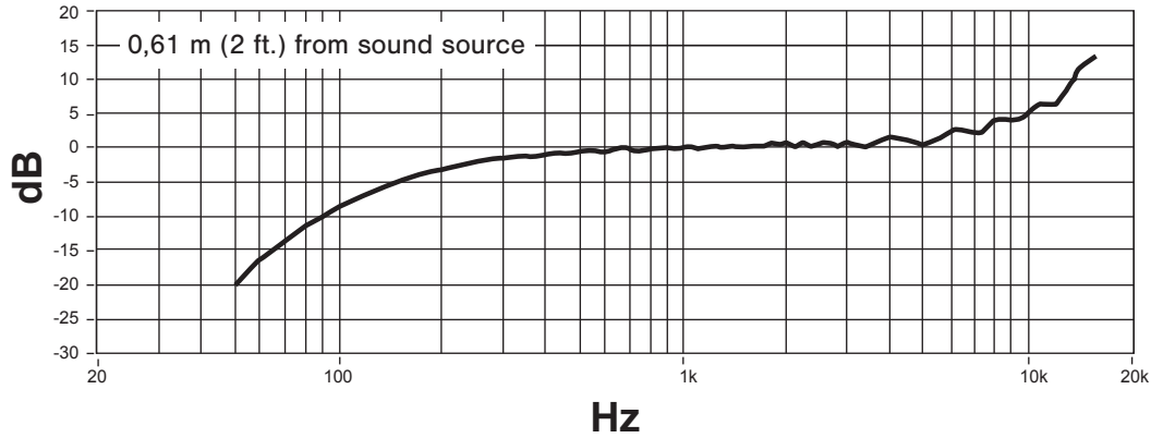
Амплитудно-частотная характеристика
