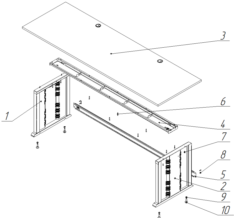
4 Схема сборки каркаса стола оператора СТО.250.80
