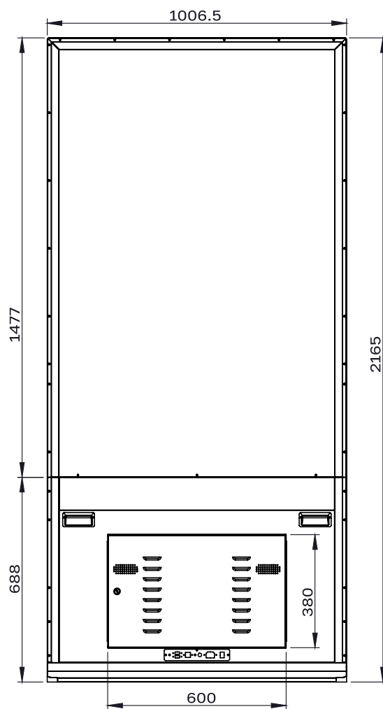
СХЕМА ДИСПЛЕЯ (ВИД СЗАДИ)
