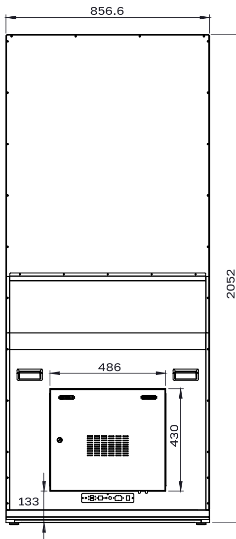
СХЕМА ДИСПЛЕЯ (ВИД СЗАДИ)
