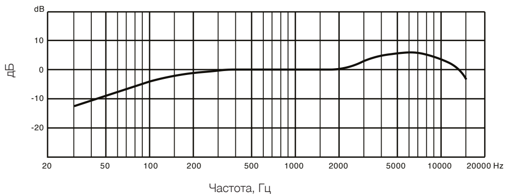
Частотный диапазон
