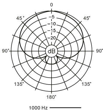
Диаграмма направленности
