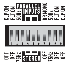
Typischer Betriebsartenschalter-Block bei Betrachtung von der Rückseite des Verstärkers (im Bild: Modell CX404V).
